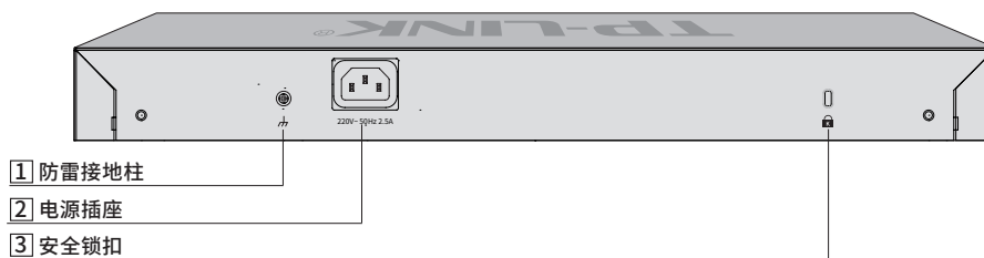
图1-8 TL-SH6428P后面板示意图
